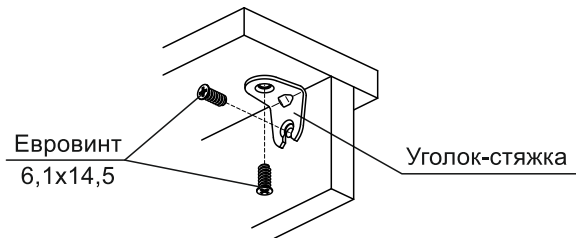
Схема 2. Установка уголка-стяжки
