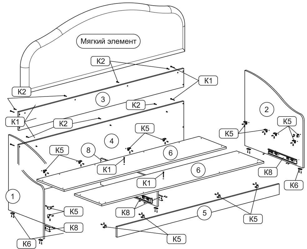
Схема 4. Сборка кровати
